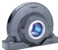
Base de línea M, de cuatro tornillos 3 3 / 16 "/80mm a 6"/155mm En hierro nodular
